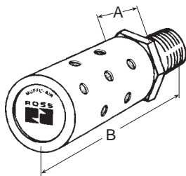
Rosca macho (según ISO 7/1-R) R 1/8 a 1-1/4
