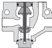
3/2 normalmente cerrada
