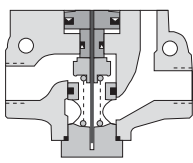
2/2 normalmente abierta
