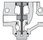
3/2 normalmente abierta
