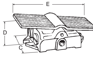
Doble Pedal
