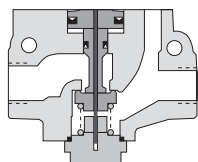
2/2 normalmente cerrada
